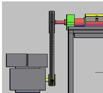
Gambar 6. Perangkaian Unit Transmisi Puly Dan Belt
