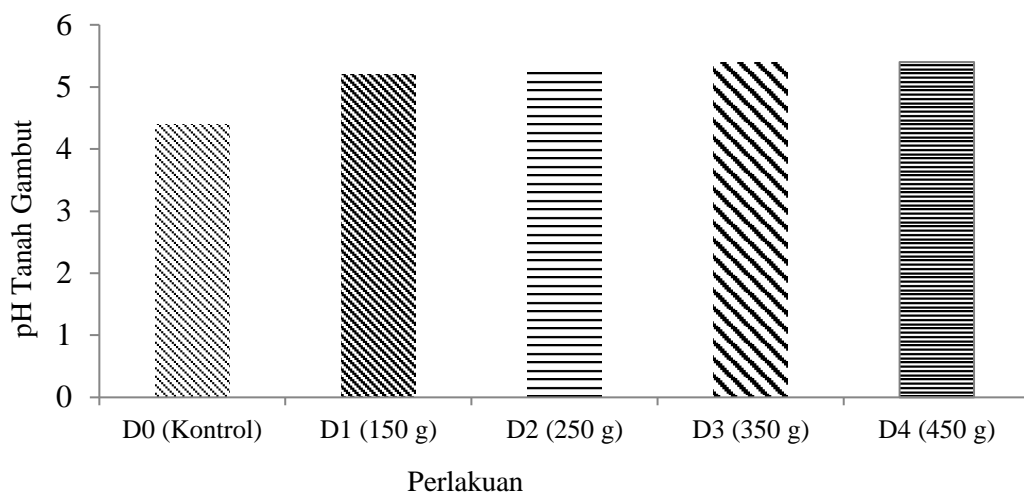
Gambar 1. pH tanah gambut akibat pengaruh pemberian abu janjang kosong kelapa sawit
